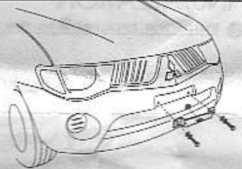
ภาพการติดตั้ง CENTER BRACKET ใต้ตัวรถ (CB-730)
