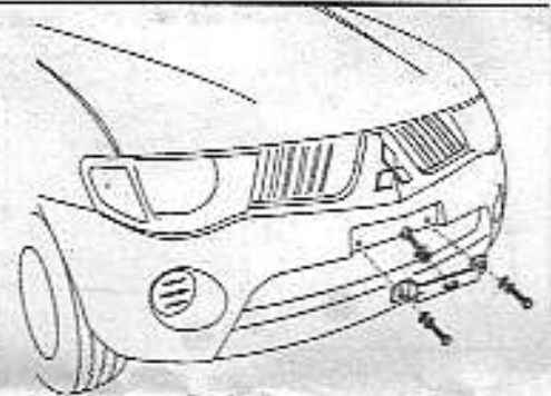
ภาพการติดตั้ง CENTER BRACKET ใต้ตัวรถ (CB-544)
